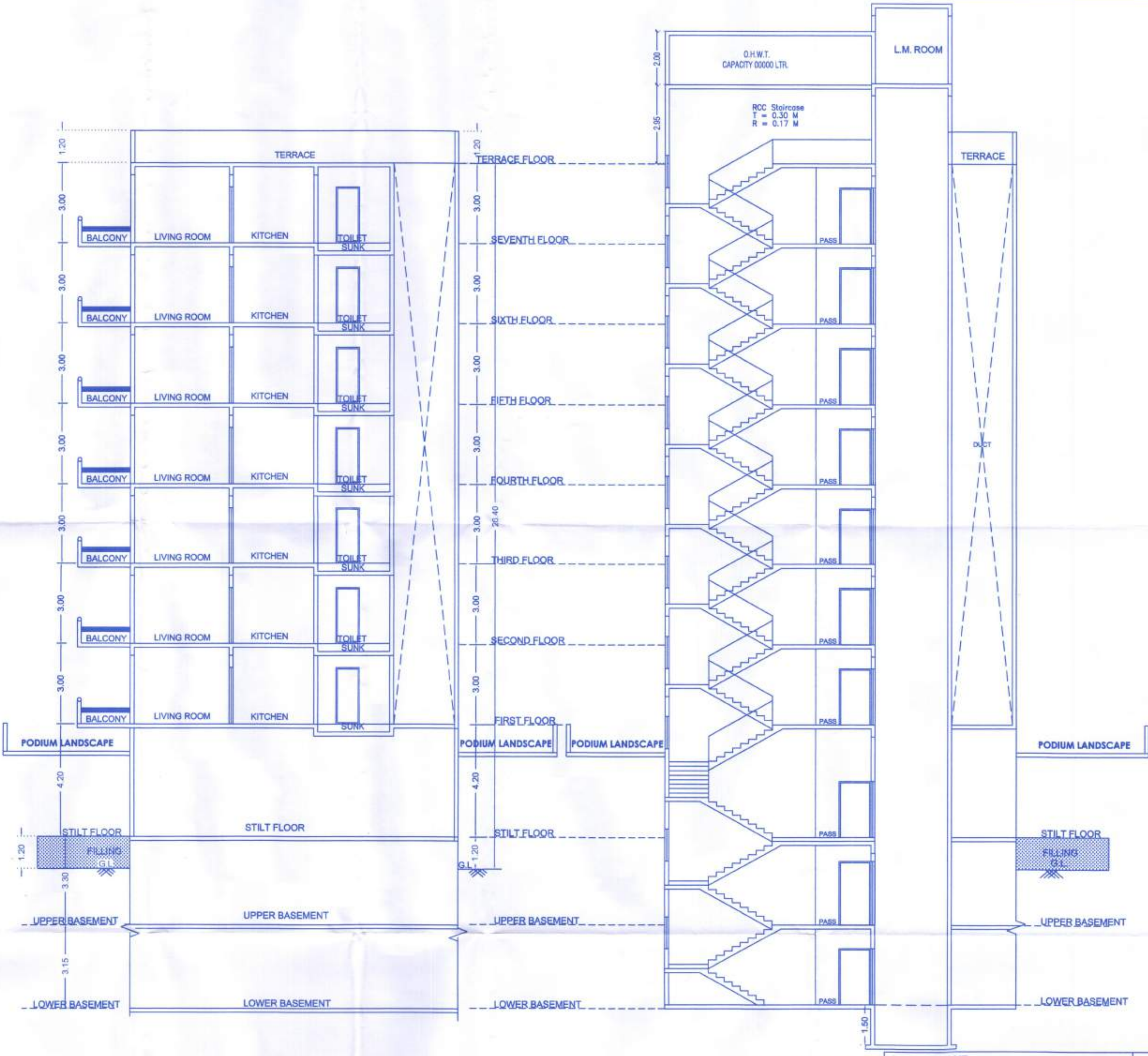
SECTION A-A
