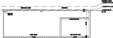
SECTION - D.D.
