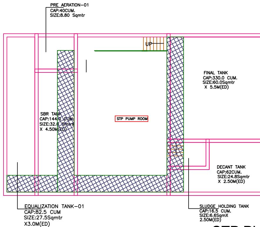
STP PLAN
