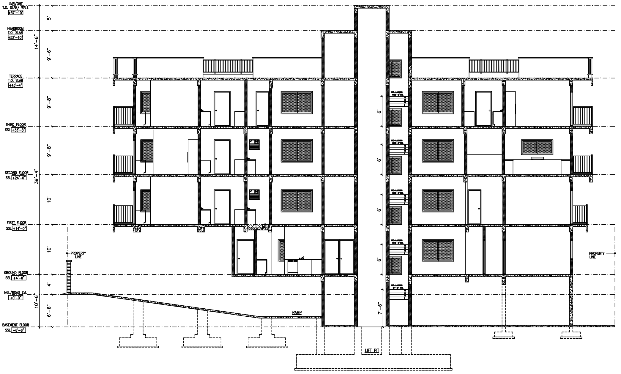
SECTION A-A
