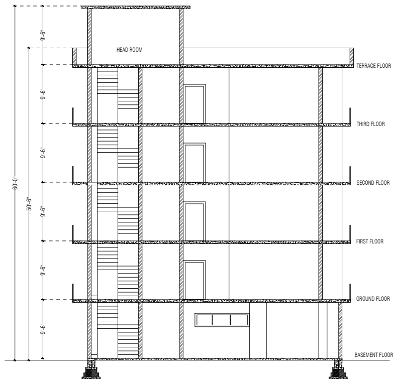
SECTION A-A
