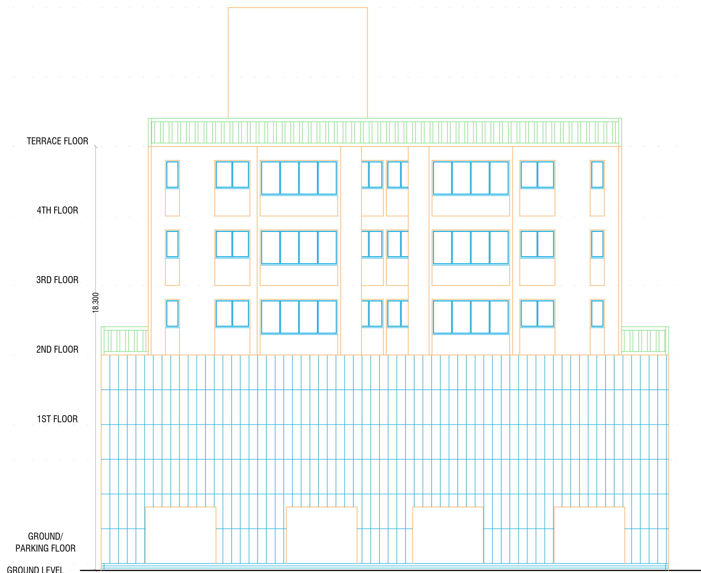
ELEVATION A
